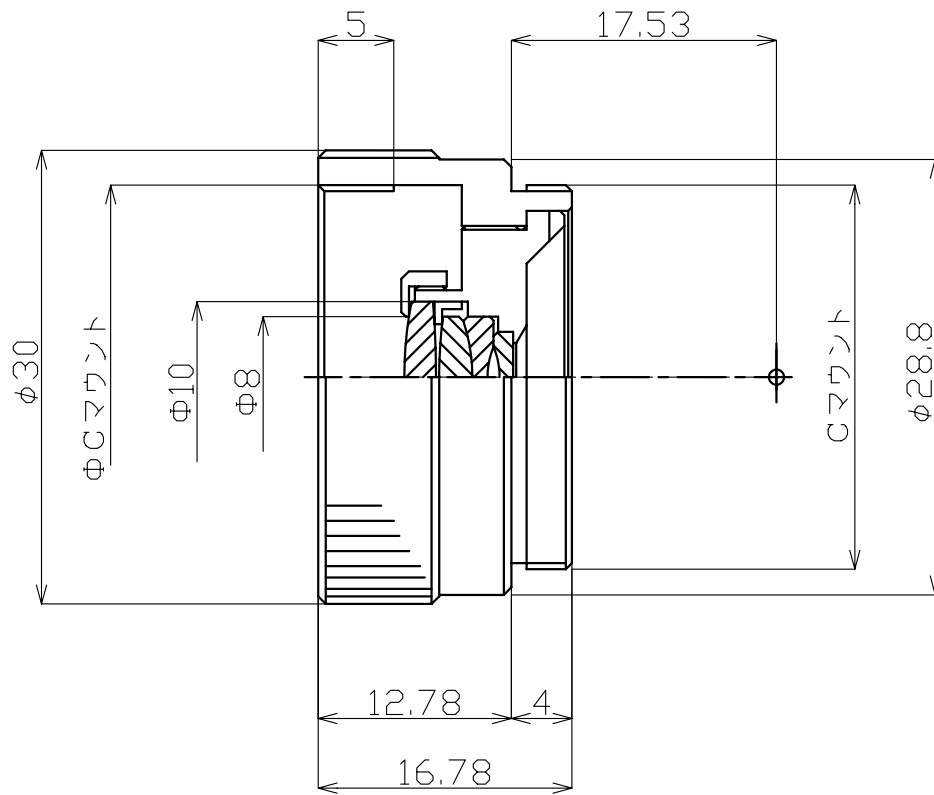
X3 リヤコンバーターレンズ
