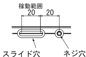
取付寸法
