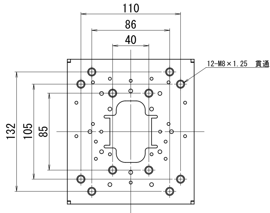
M8ネジ穴詳細図 (表面)
